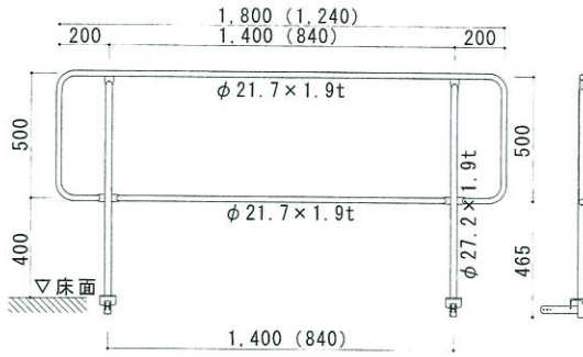
手すり取付部<差込み>タイプ
