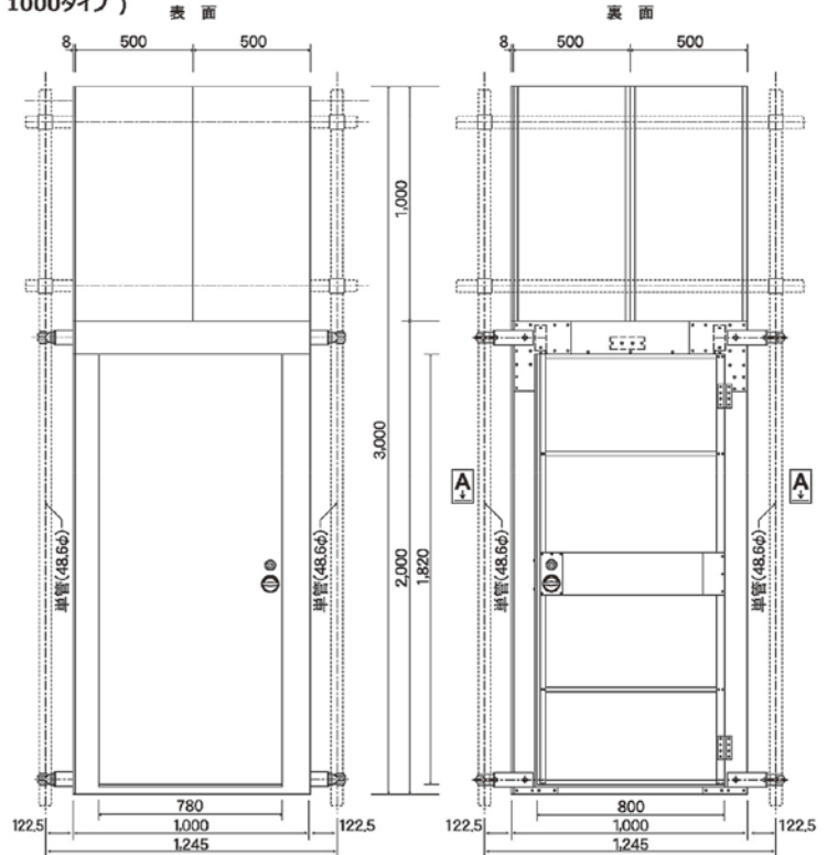
製品図 (1000タイプ)
